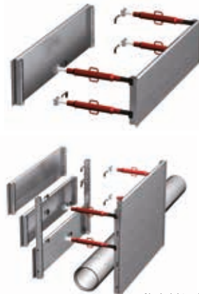
Alu-Leichtverbau GIGANT
